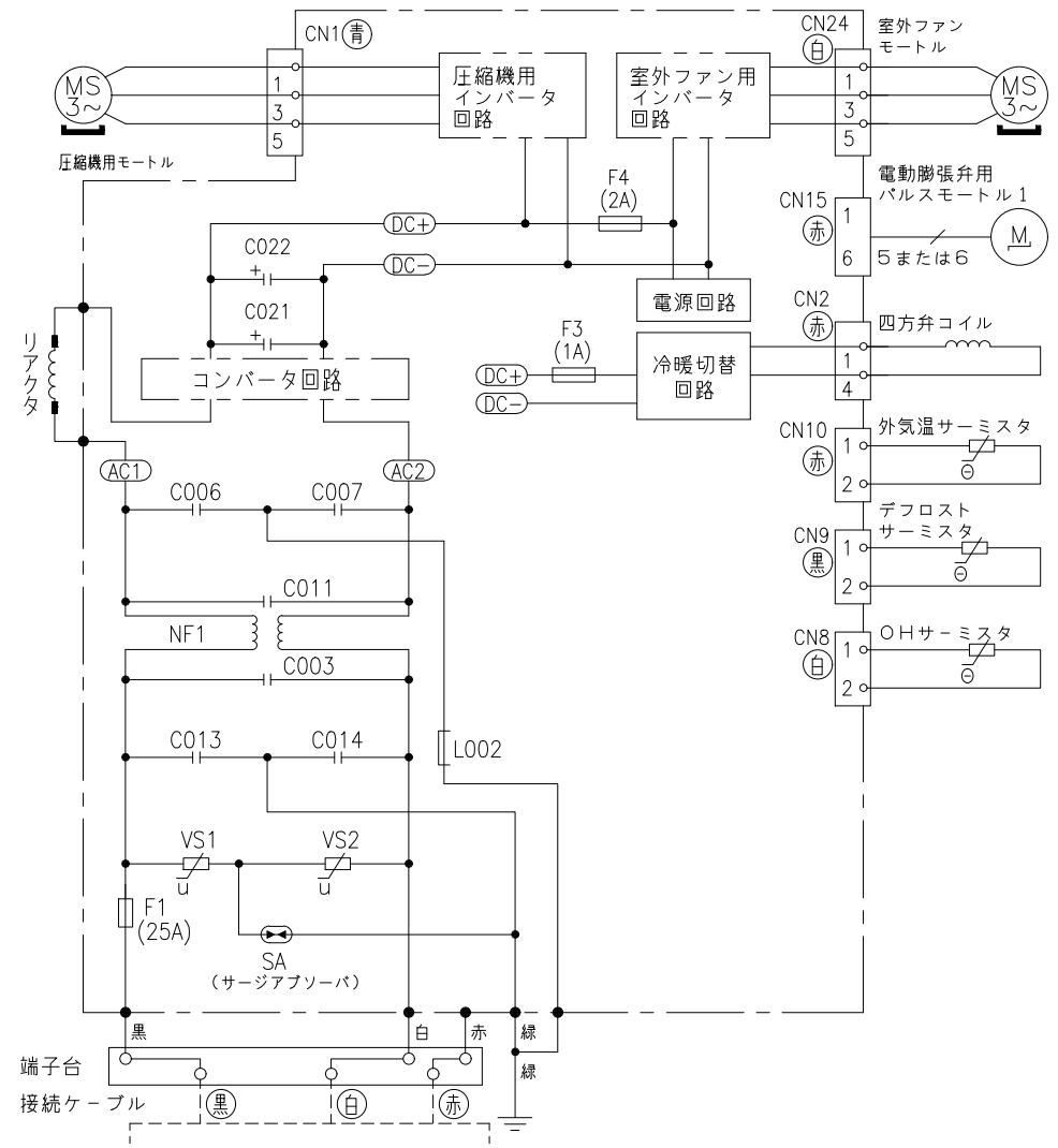
配線図 RAC-JT80K2E8
