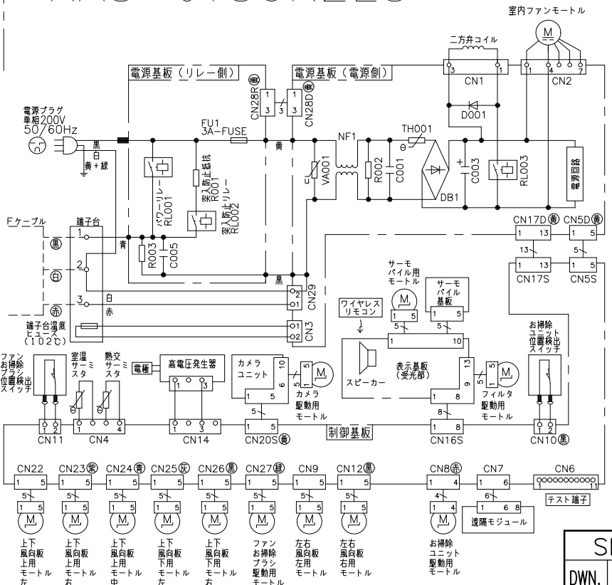
配線図 RAS-JT80K2E8
