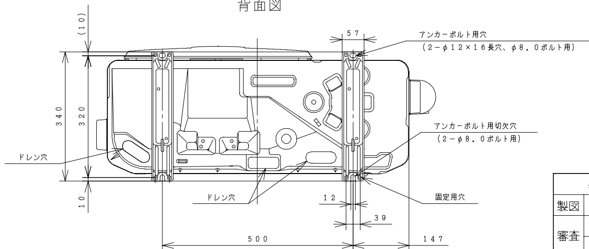
背面図
