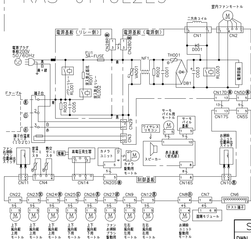
配線図 RAS-JT40L2E9
