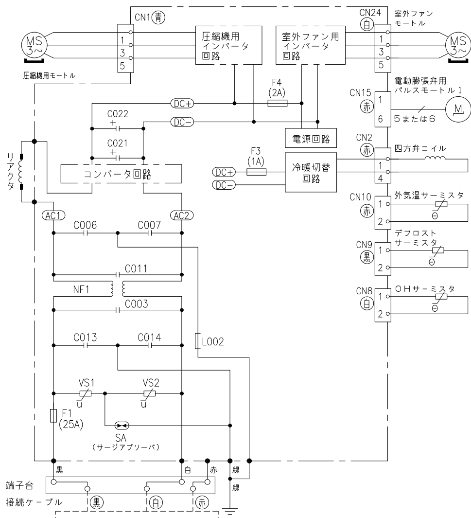
配線図 RAC-JT40L2E9
