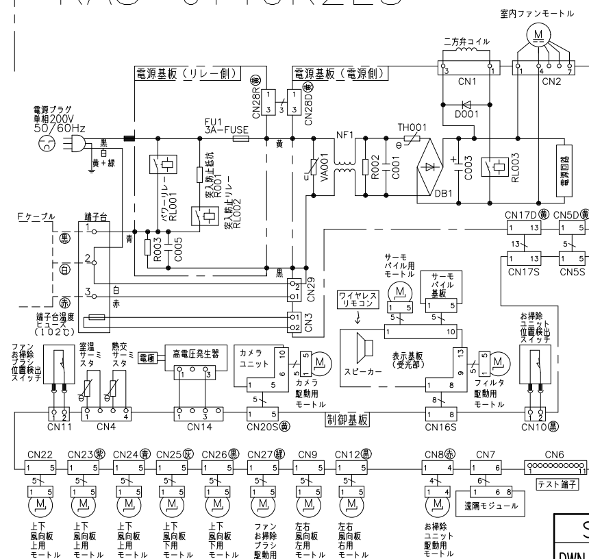
配線図 RAS-JT40K2E8
