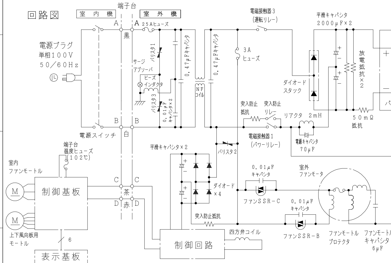
配線図 HRS-28JX
