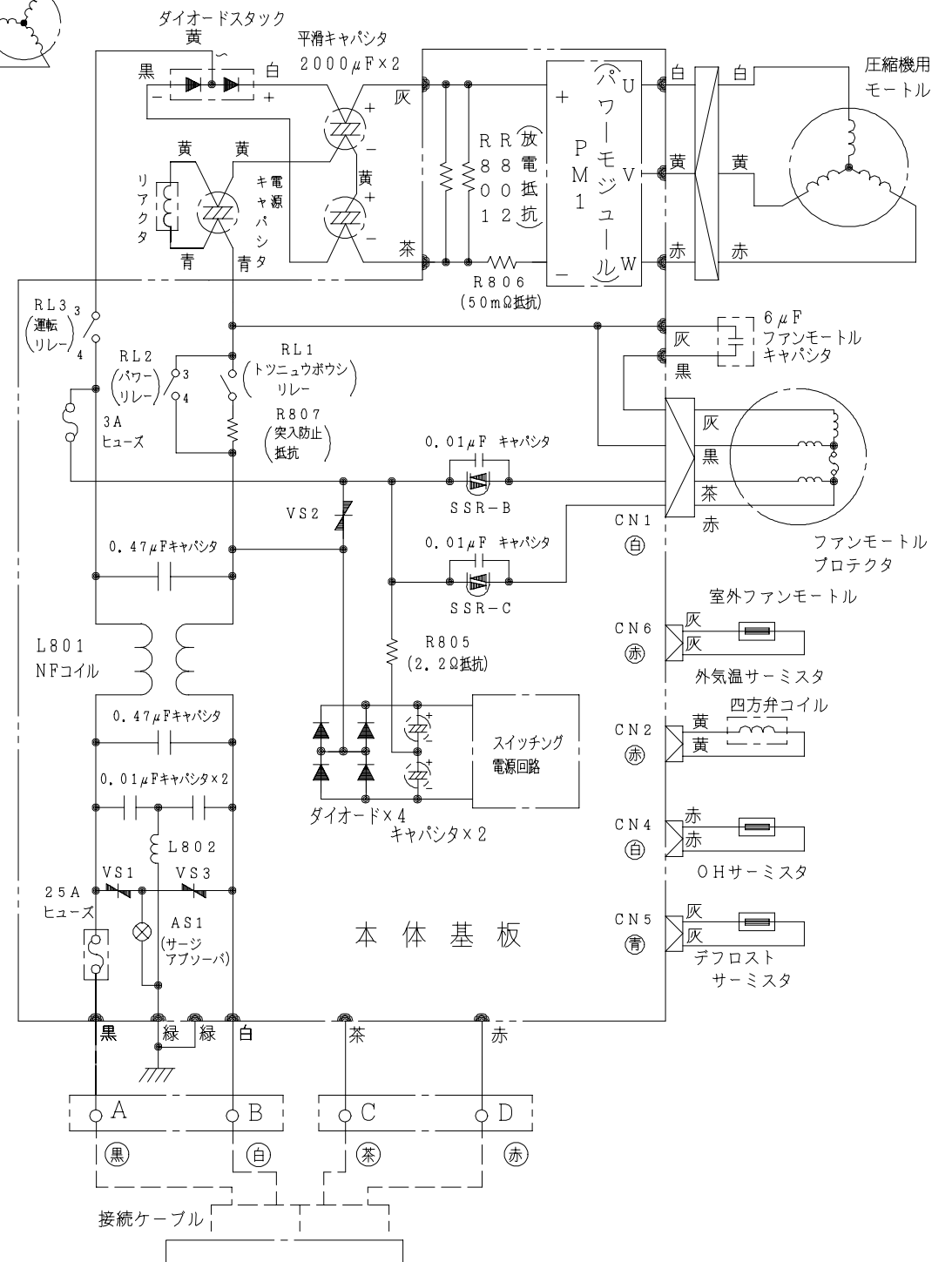
配線図 HRC-28JX
