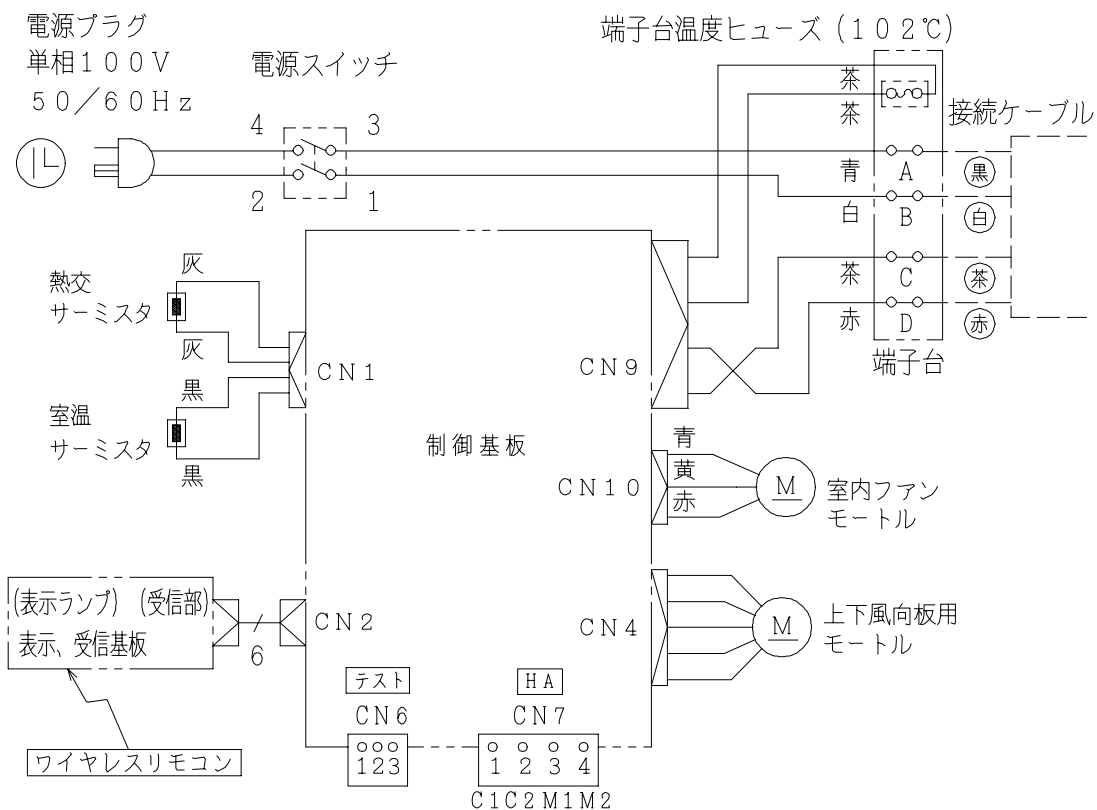
配線図 HRS-28JX
