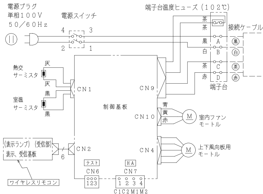
配線図 HRS-25JX
