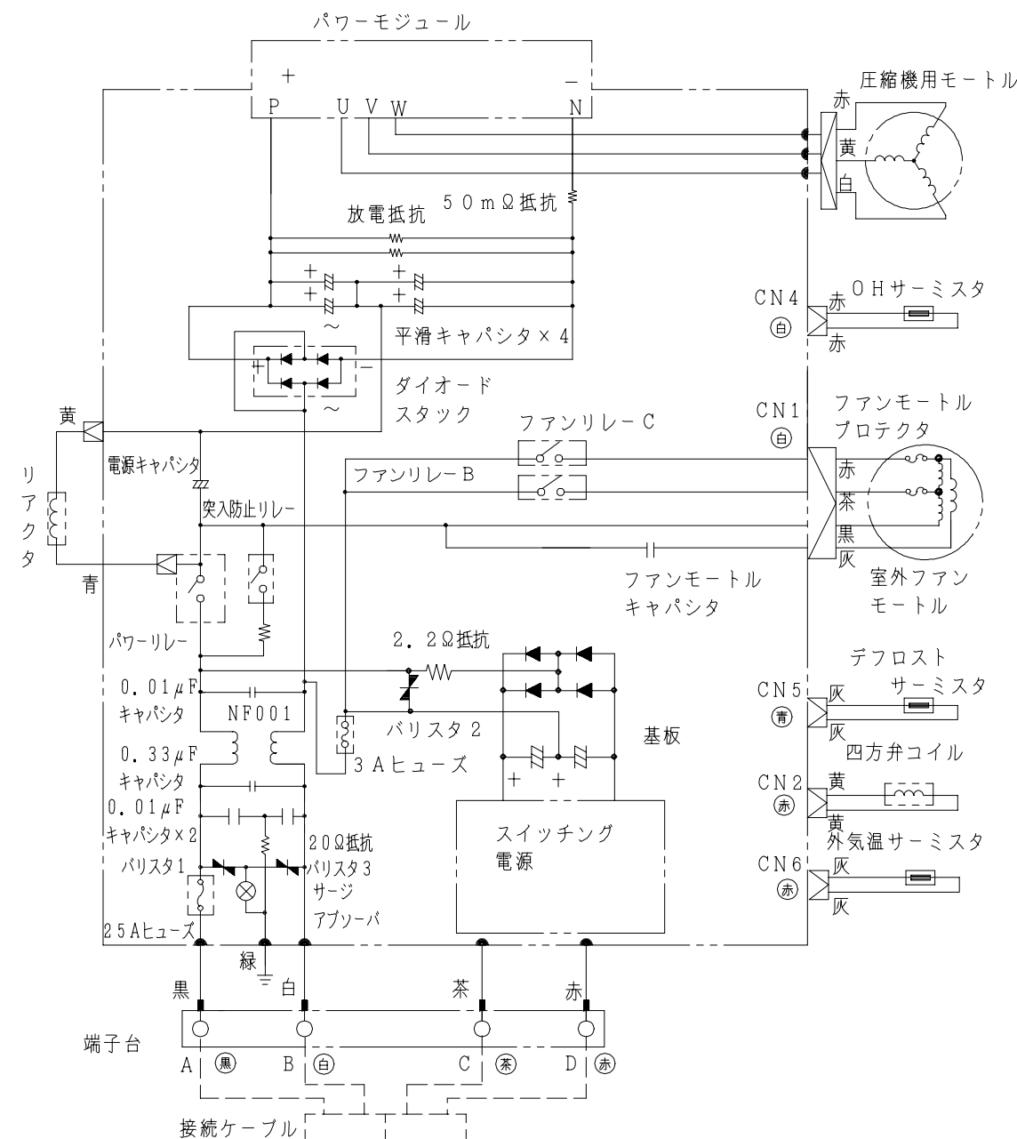
配線図 HRC-25JX
