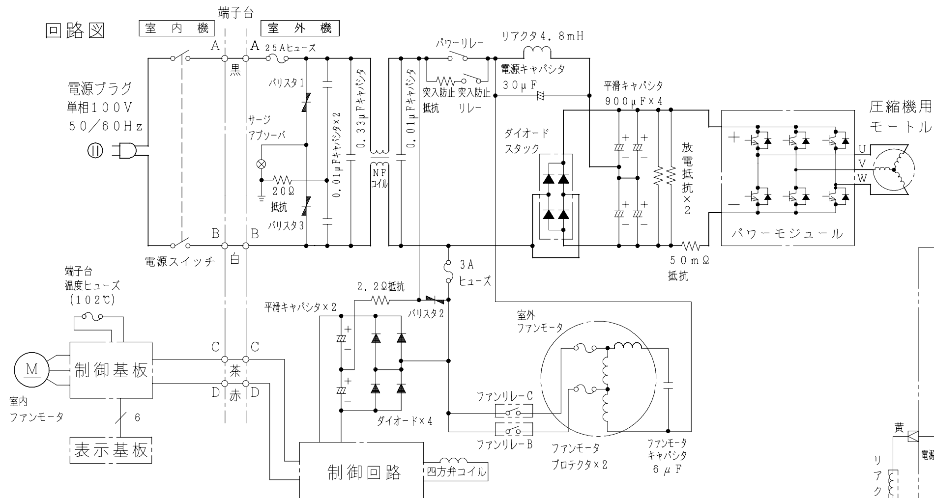
配線図 HRS-25JX
