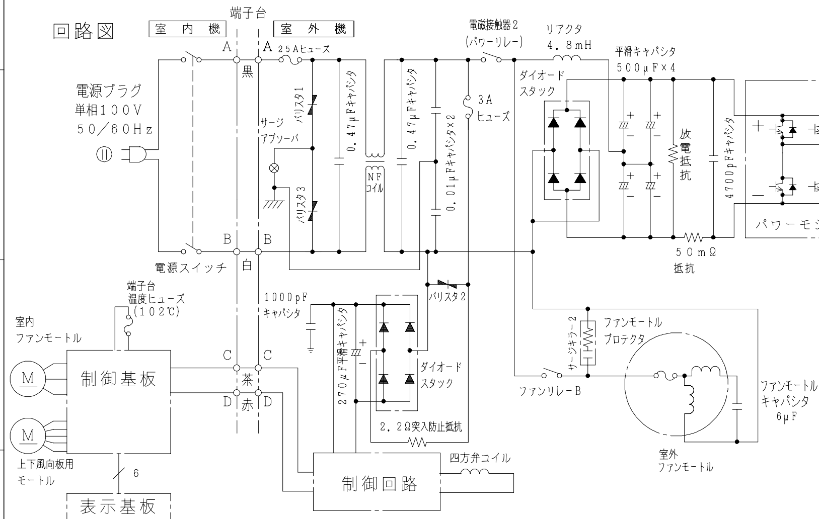
配線図 HRS-22LX
