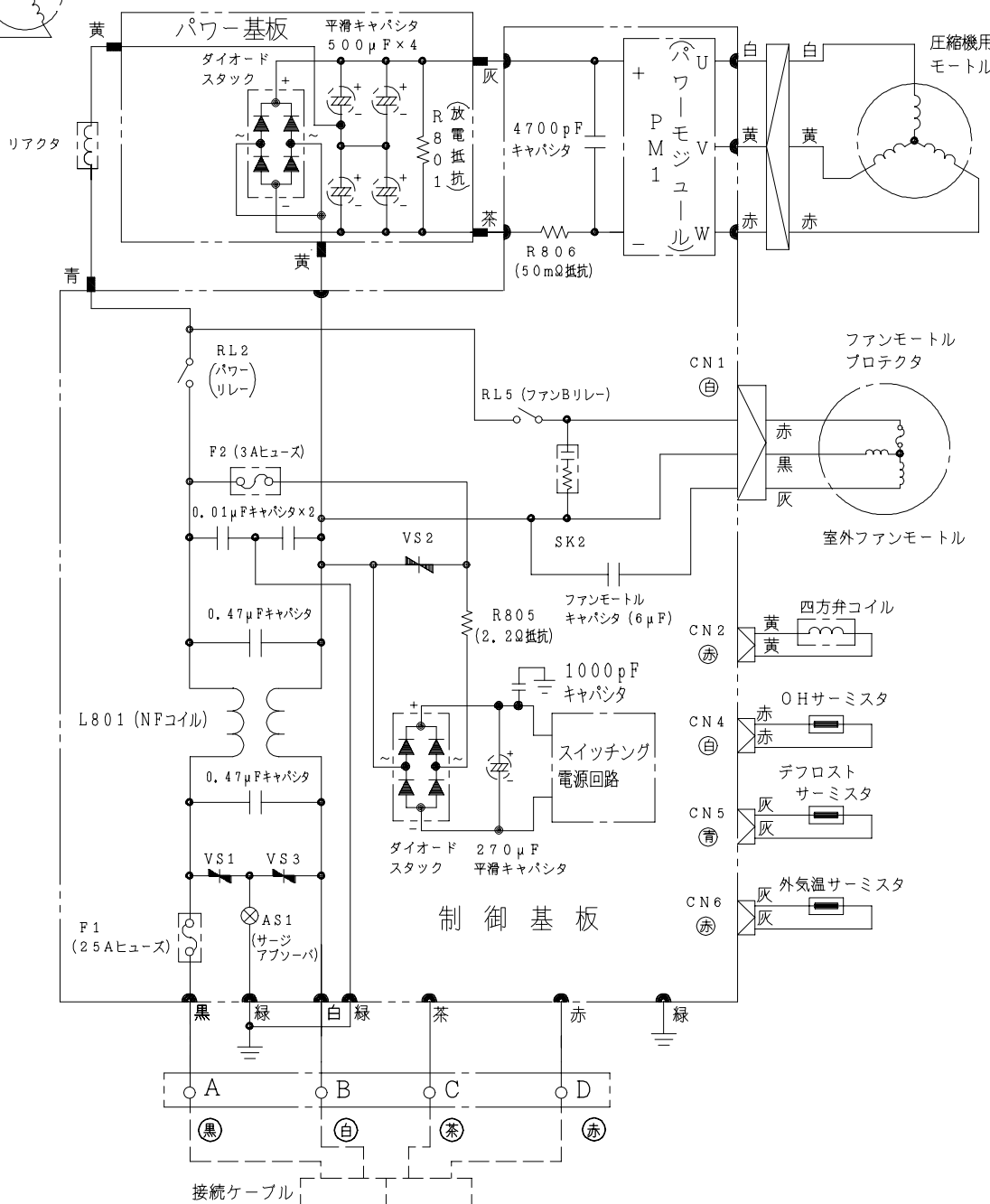
配線図 HRC-22LX
