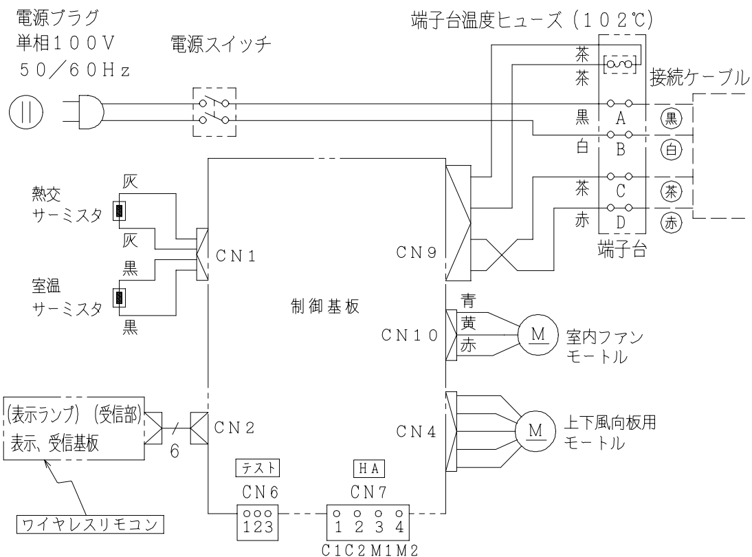
配線図 HRS-22LX
