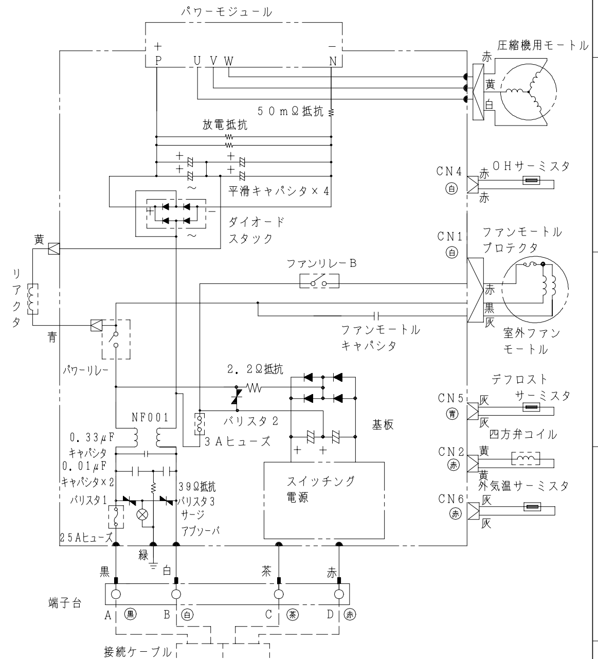
配線図 HRC-22JX-1
