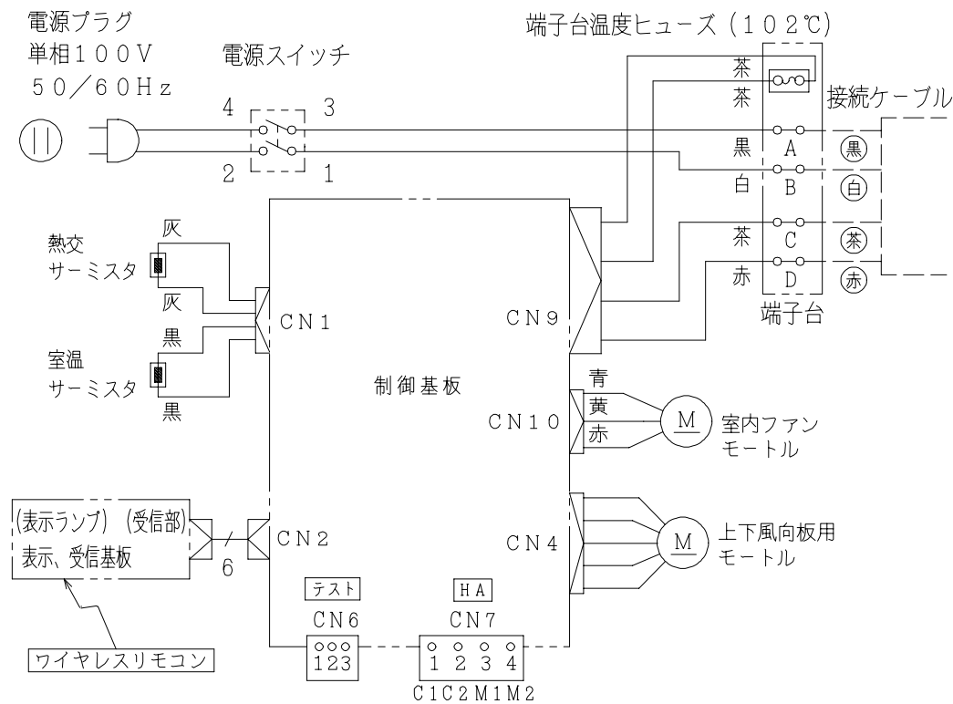
配線図 HRS-22JX-1
