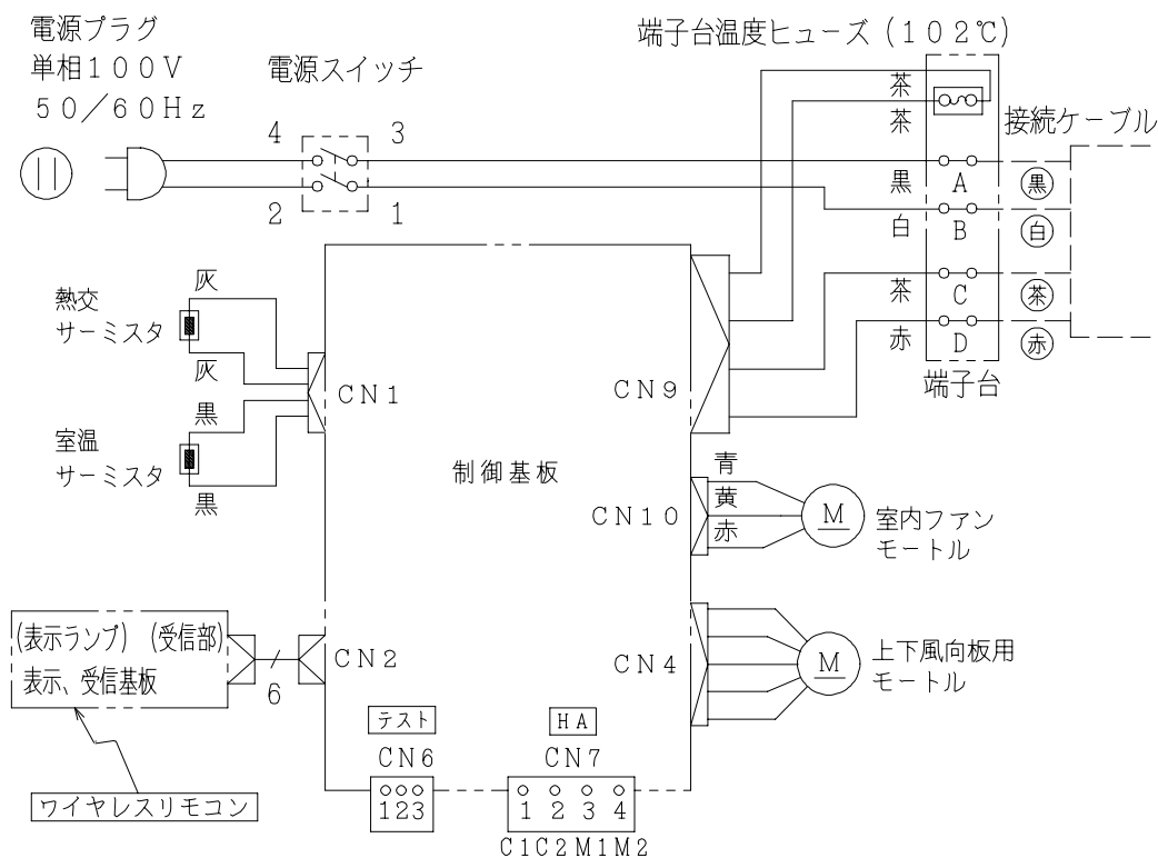
配線図 HRS-22JX
