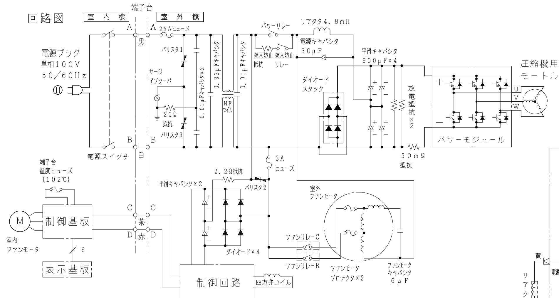
配線図 HRS-22JX
