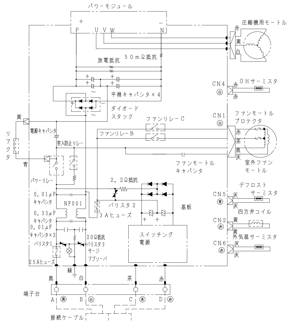
配線図 HRC-22JX
