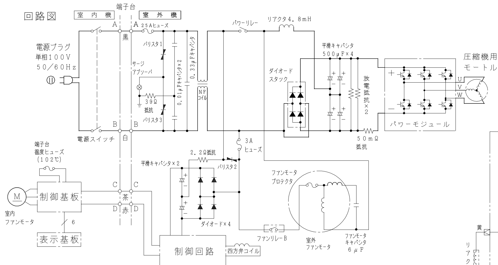
配線図 HRS-22JW-1
