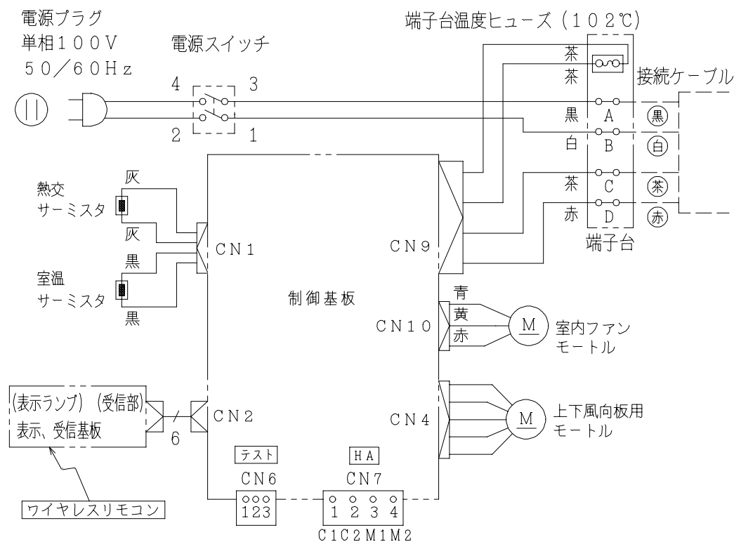
配線図 HRS-22JW-1
