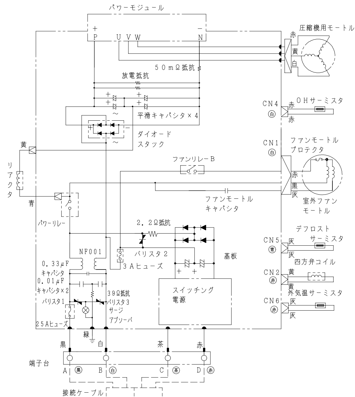
配線図 HRC-22JW-1
