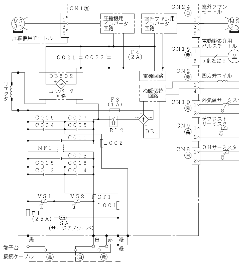
配線図 R A C - E H 4 0 H 2 E 6
