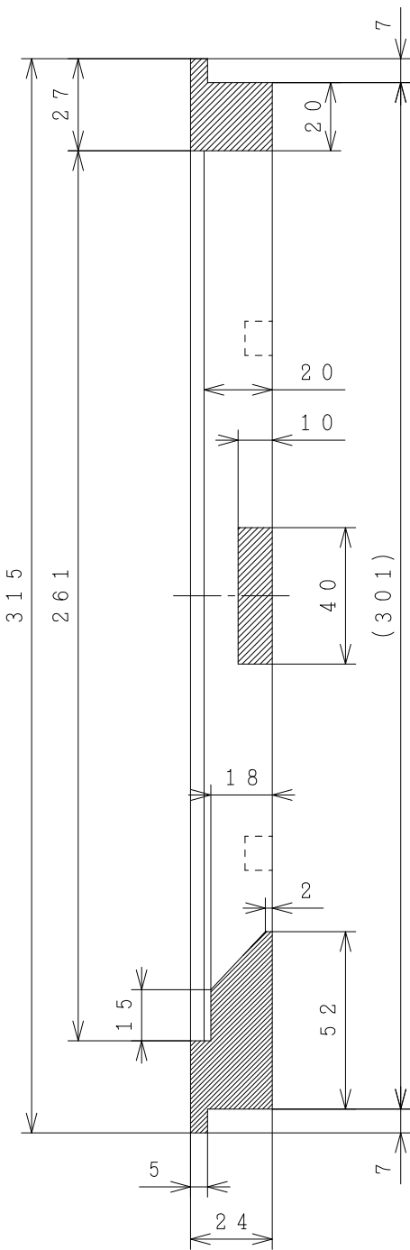
B-B' 断面図
