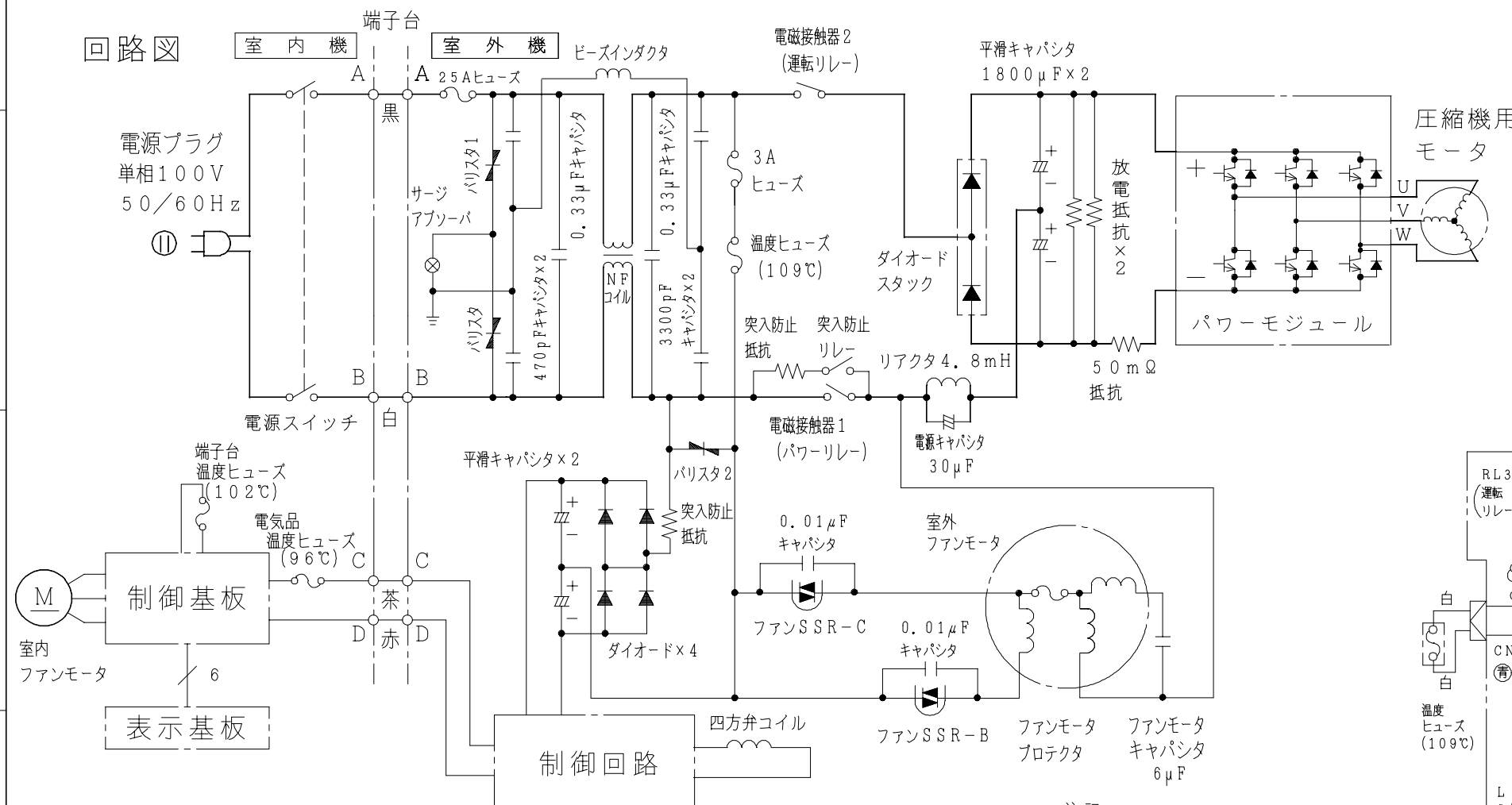
配線図 CRS-A25FX
