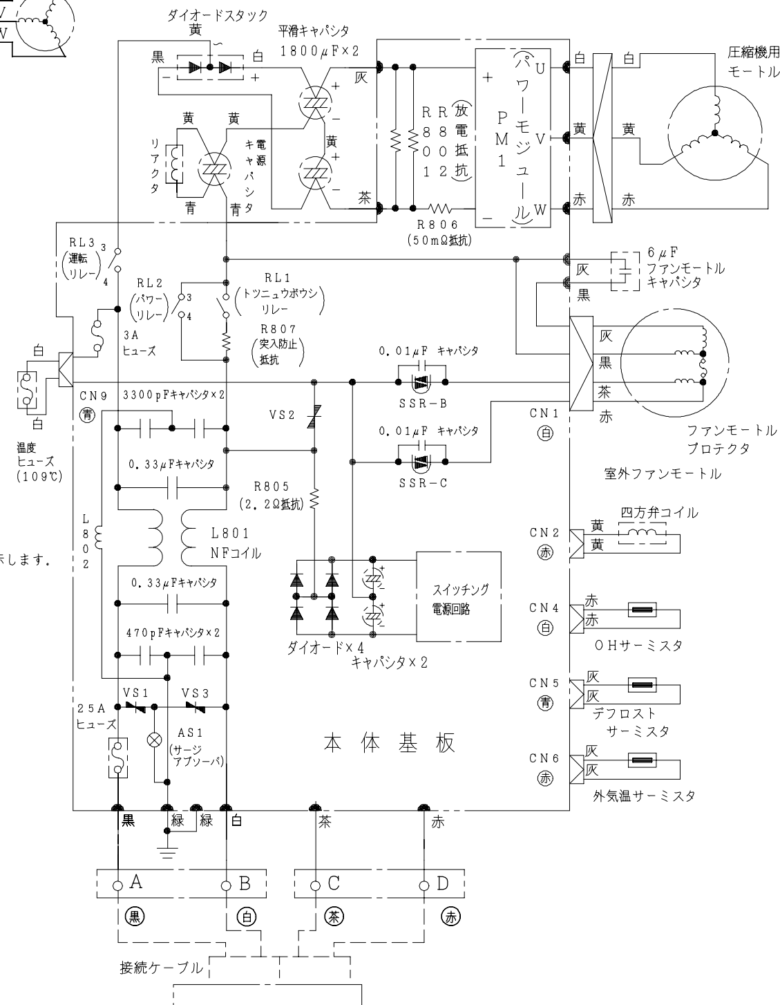
配線図 CRS-A25FX
