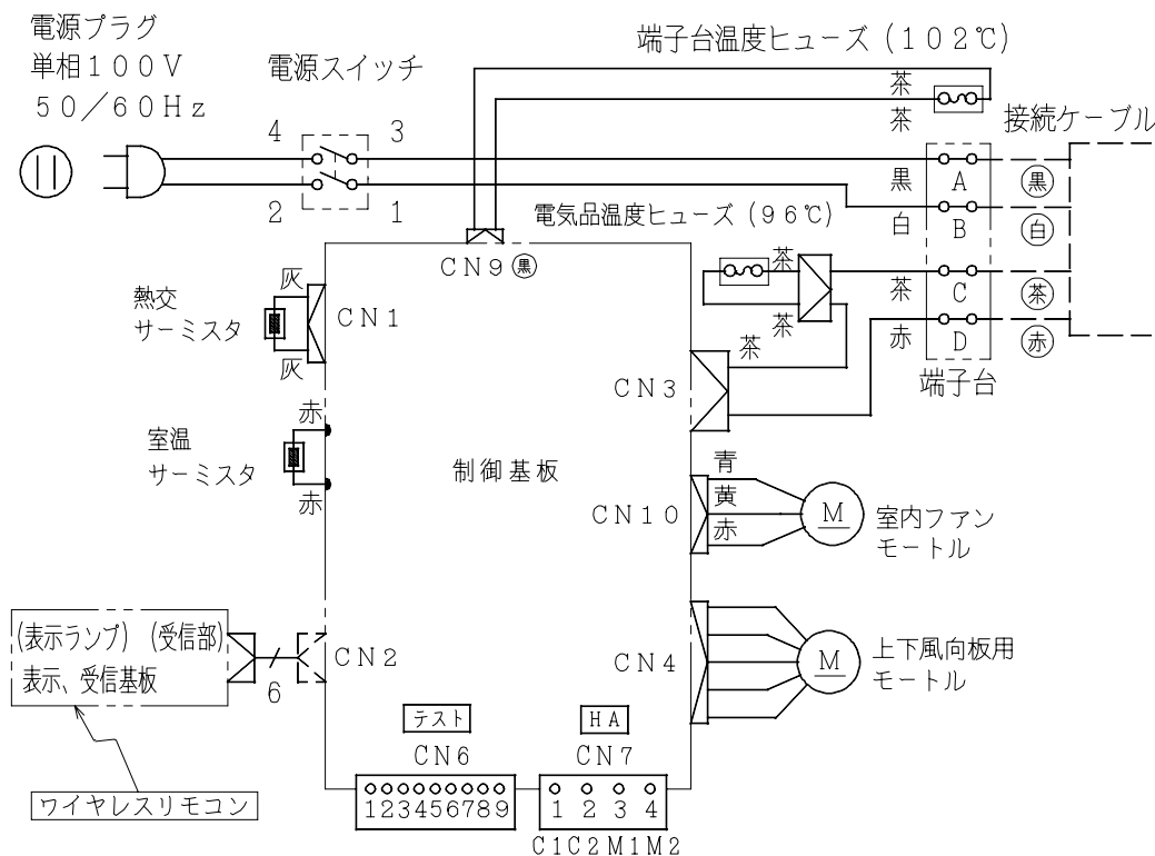
配線図 CRS-A25FX
