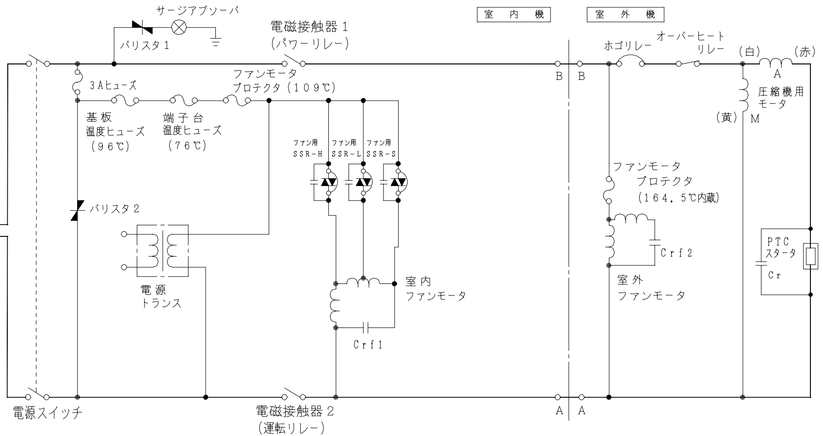
回路図
