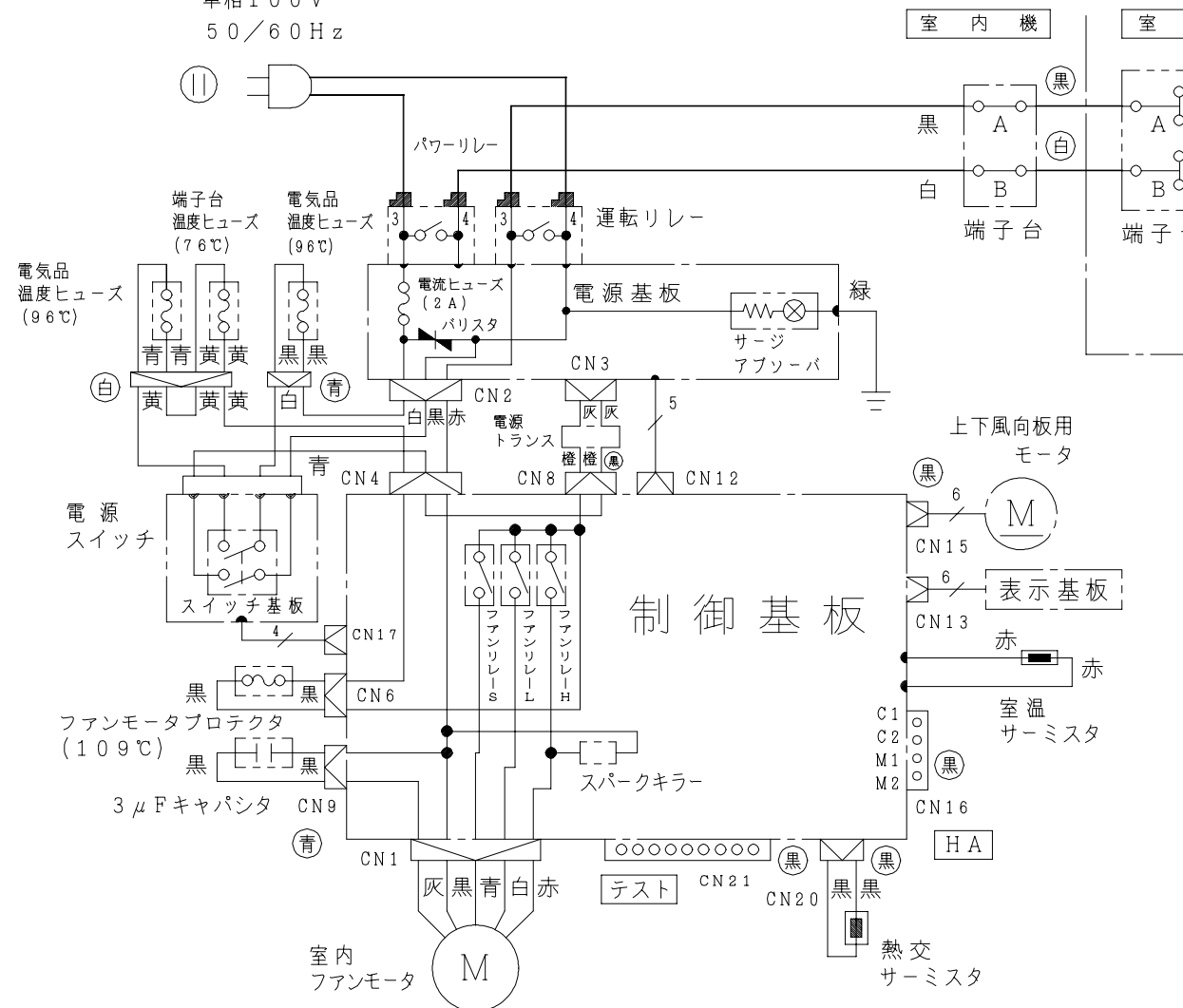
配線図
