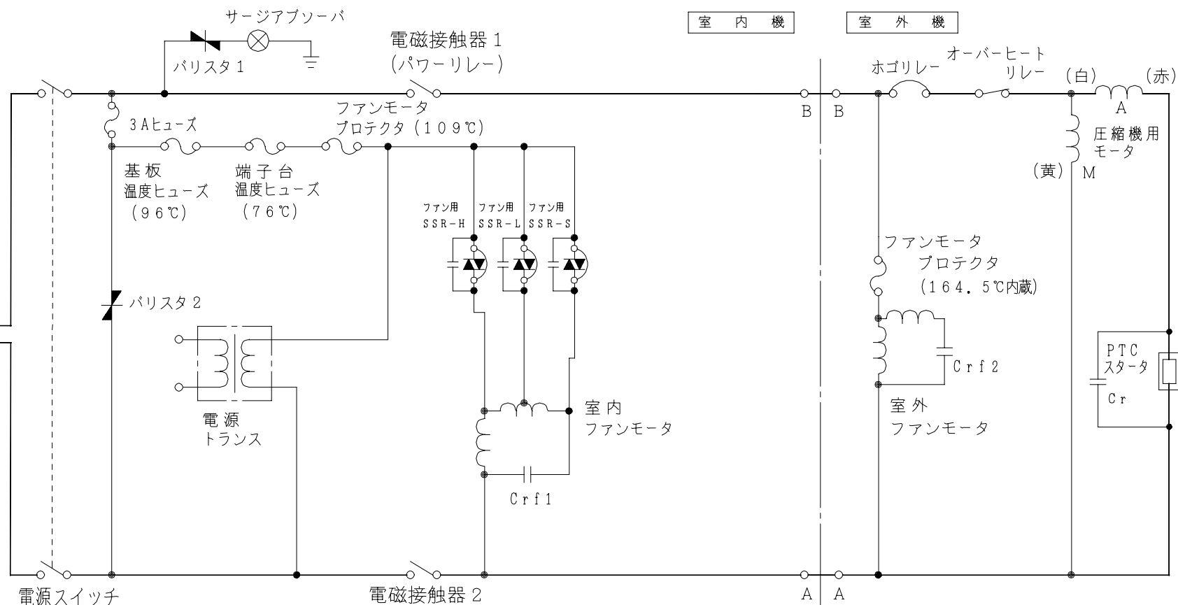
回路図
