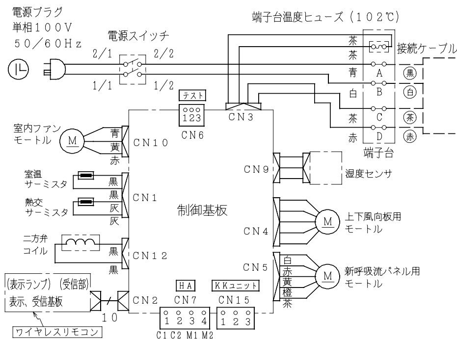
配線図 RAS-2810JX
