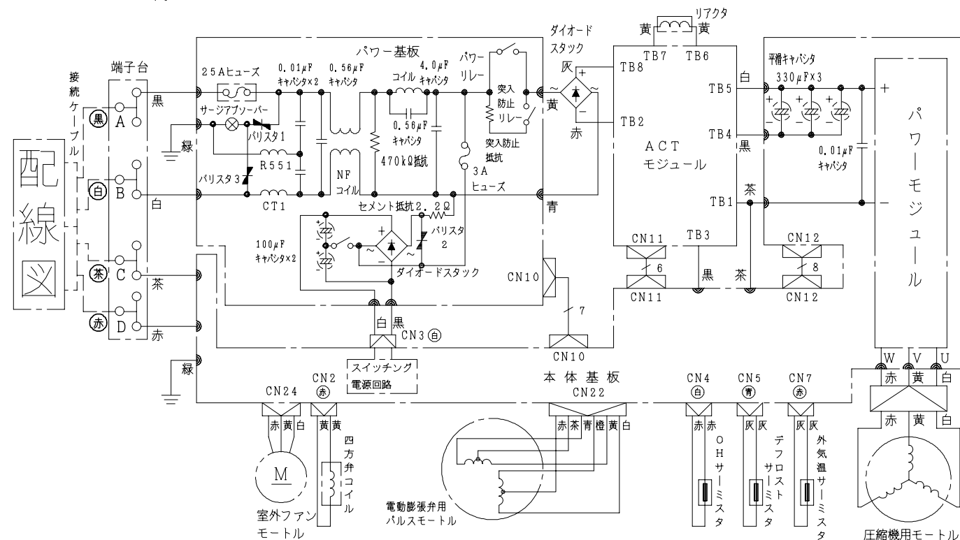
配線図 RAC-2810JX-1
