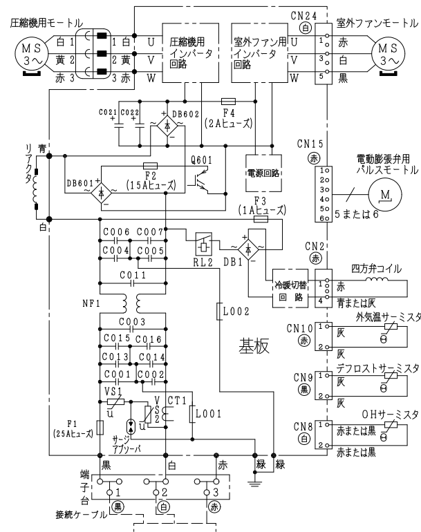
配線図 R A C - Z J 6 3 F 2
