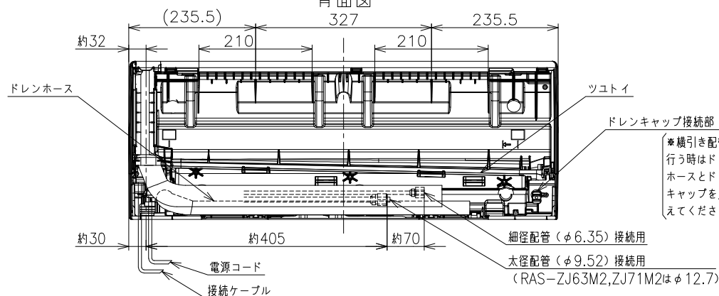
背面図
