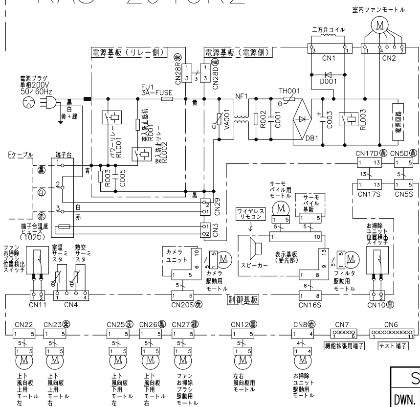
配線図 RAS-ZJ40K2
