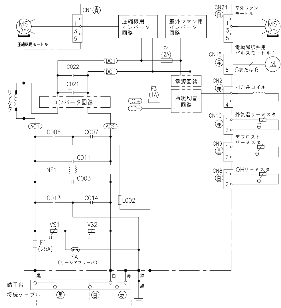
配線図 RAC-ZJ40K2
