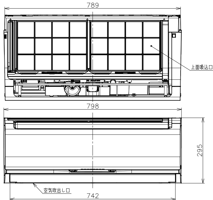
日立ルームエアコン 壁掛ZJEシリーズ 室内ユニット 寸法図
