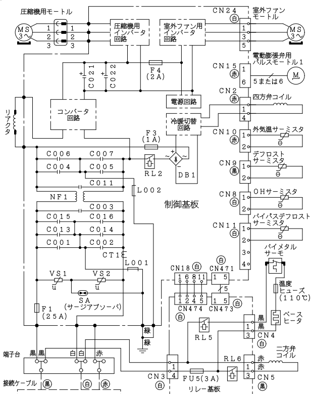
配線図 R A C - X K 6 3 H 2
