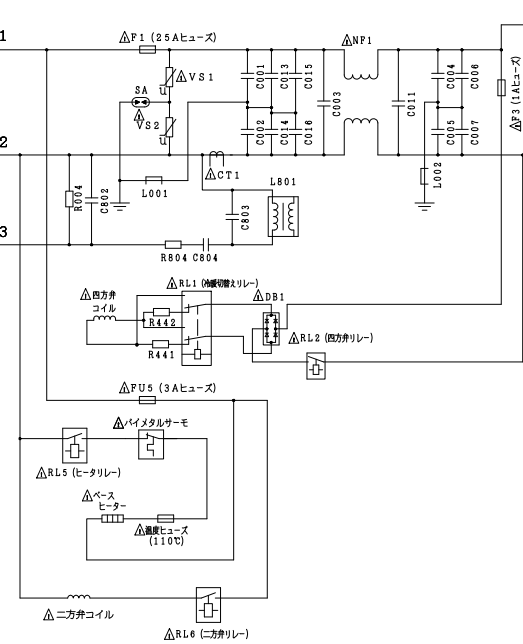
配線図 RAS-XK63H2
