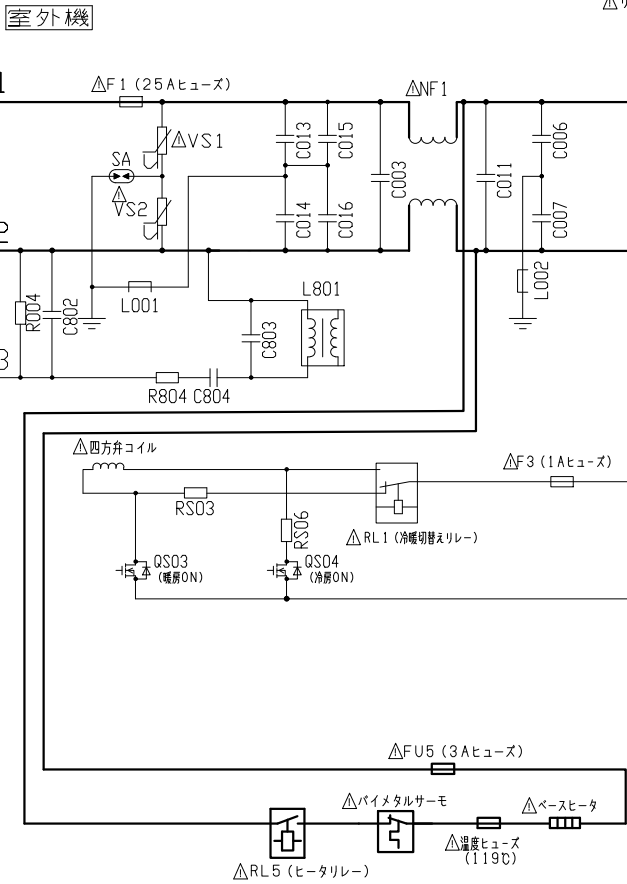
配線図 RAS-XK56L2
