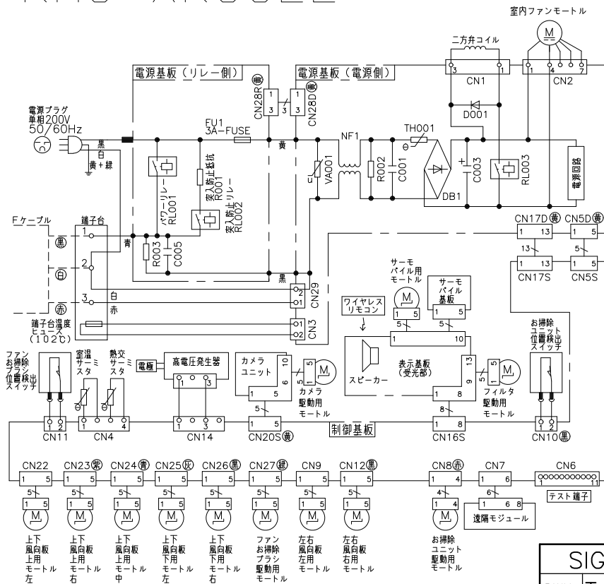
配線図 RAS-XK56L2
