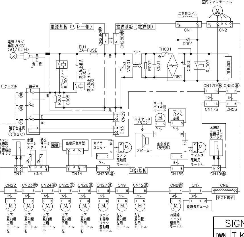
配線図 RAS-XK28L2
