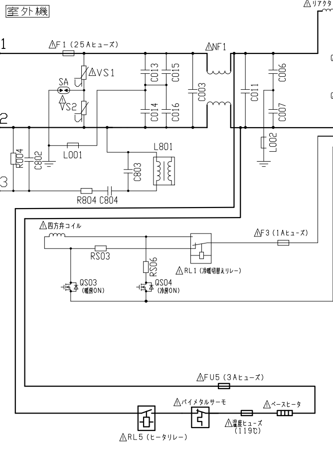
配線図 RAS-XK28L2
