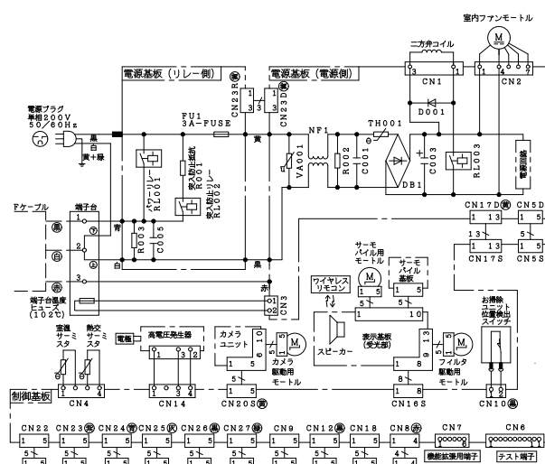
配線図 RAS-XJ90H2
