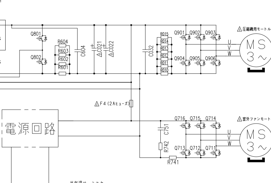
配線図 RAC-XJ63K2
