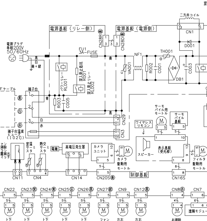
配線図 RAS-XJ63K2
