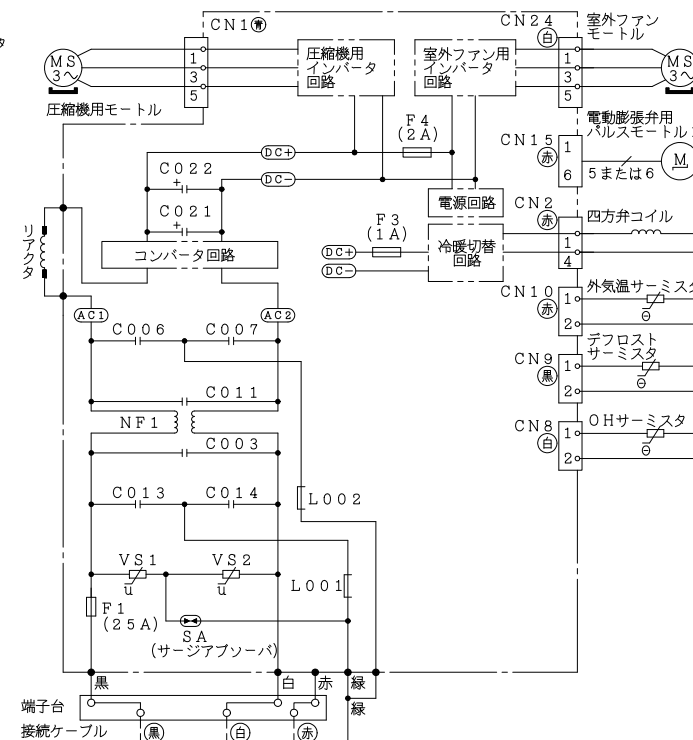
配線図 R A C - X J 6 3 J 2
