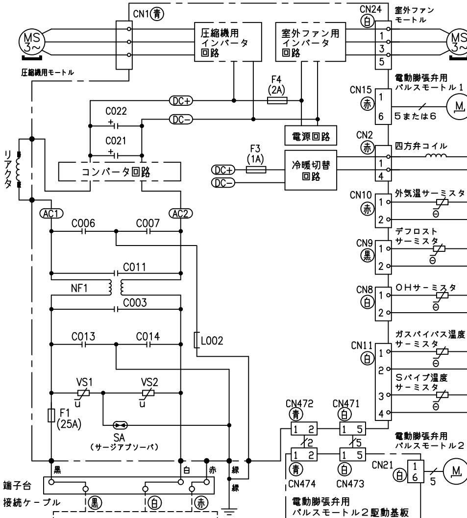
配線図 RAC-XC90L2
