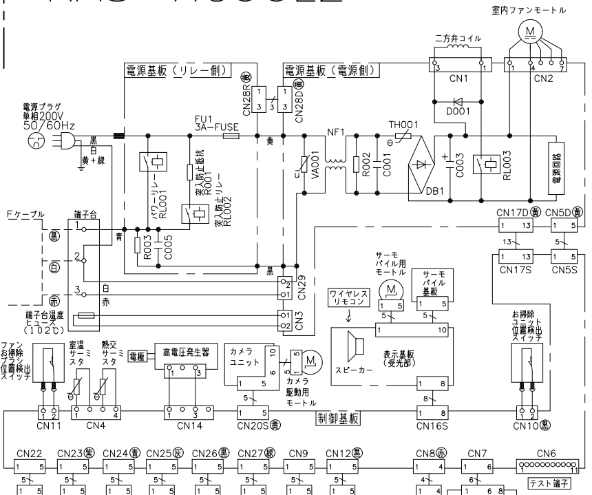
配線図 RAS-XC90L2
