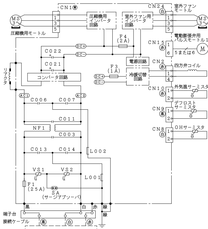
配線図 R A C - X C 8 0 J 2
