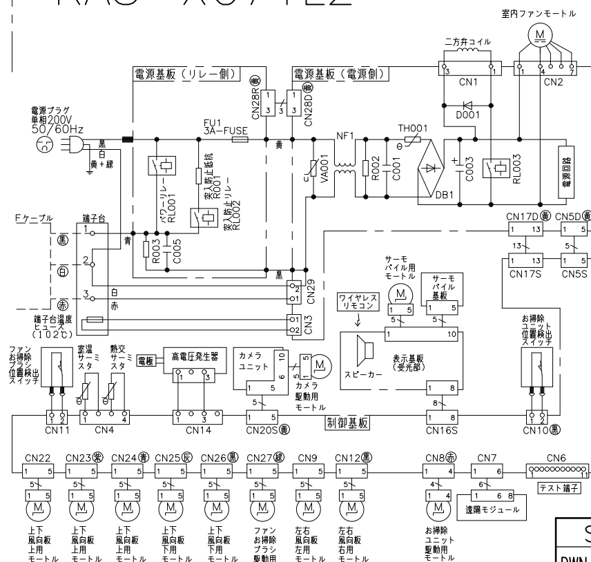
配線図 RAS-XC71L2
