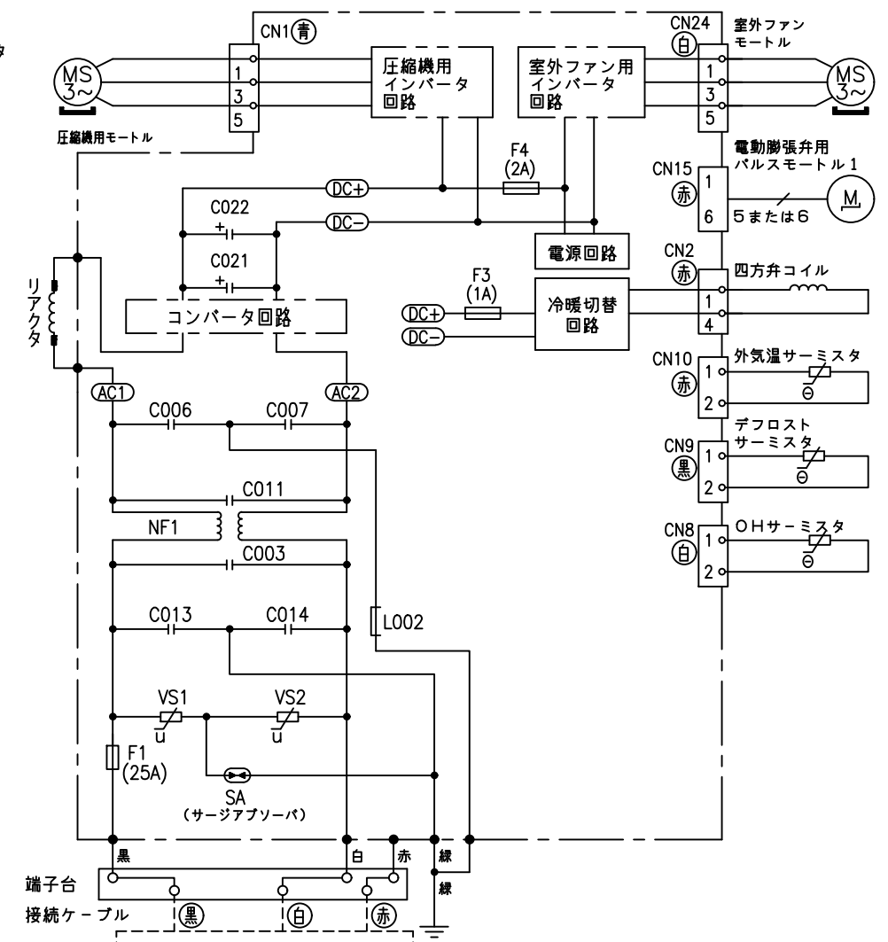
配線図 RAC-XC71L2
