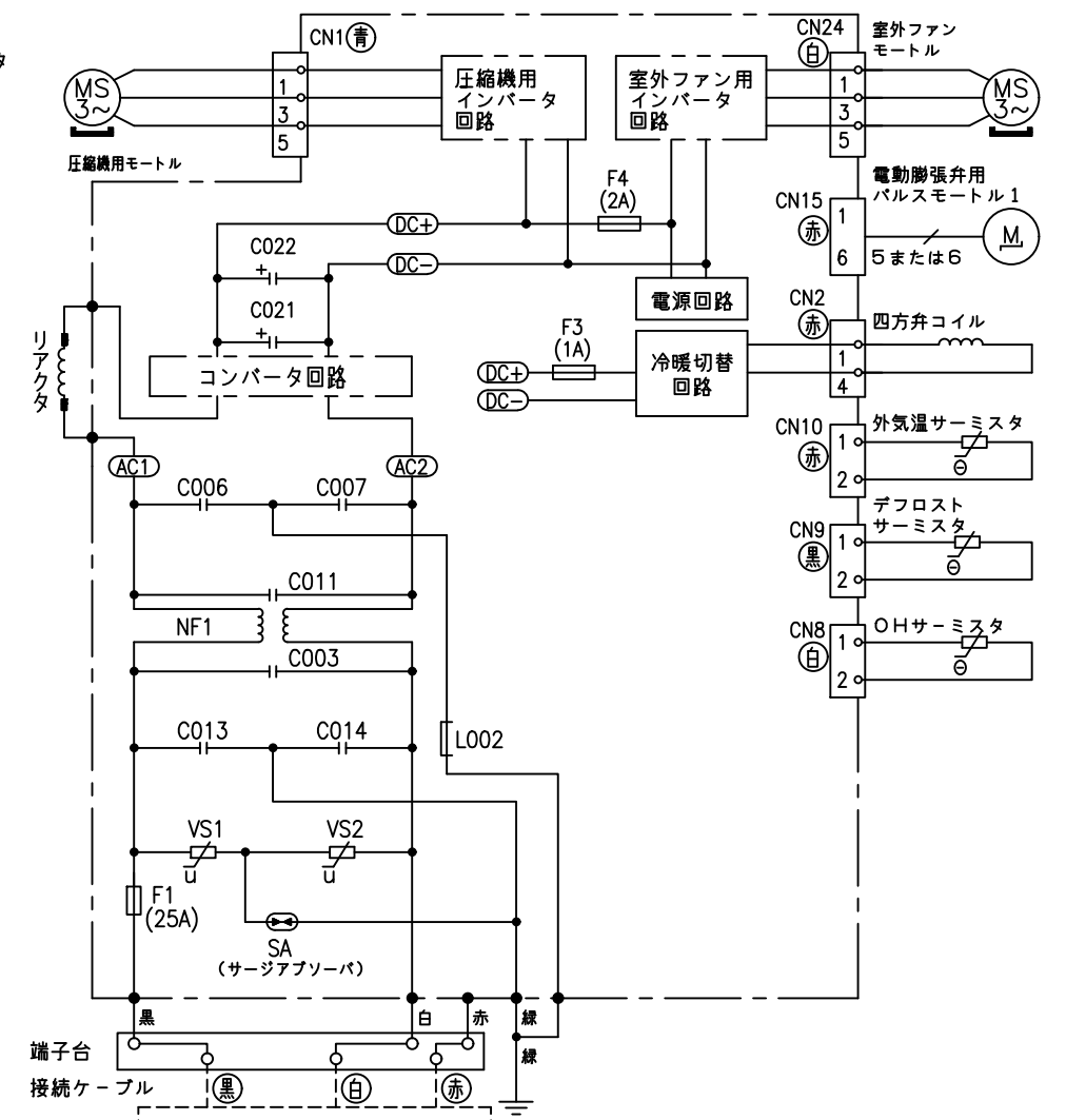
配線図 RAC-XC71K2
