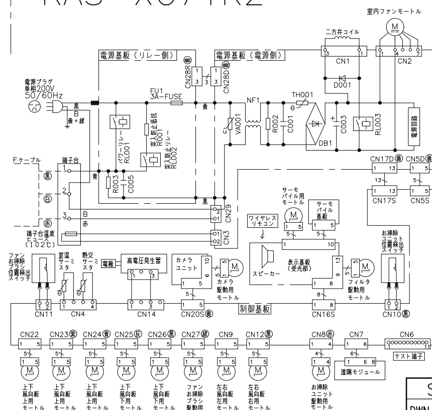
配線図 RAS-XC71K2
