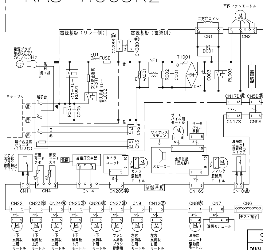
配線図 RAS-XC63K2
