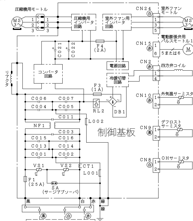
配線図 R A C - X C 5 6 F 2
