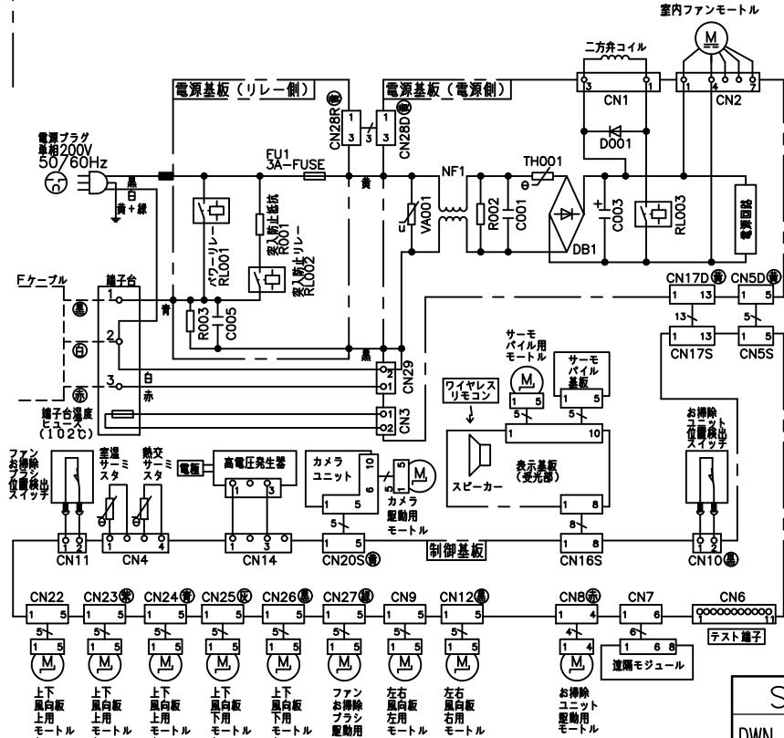
配線図 RAS-XC36L2
