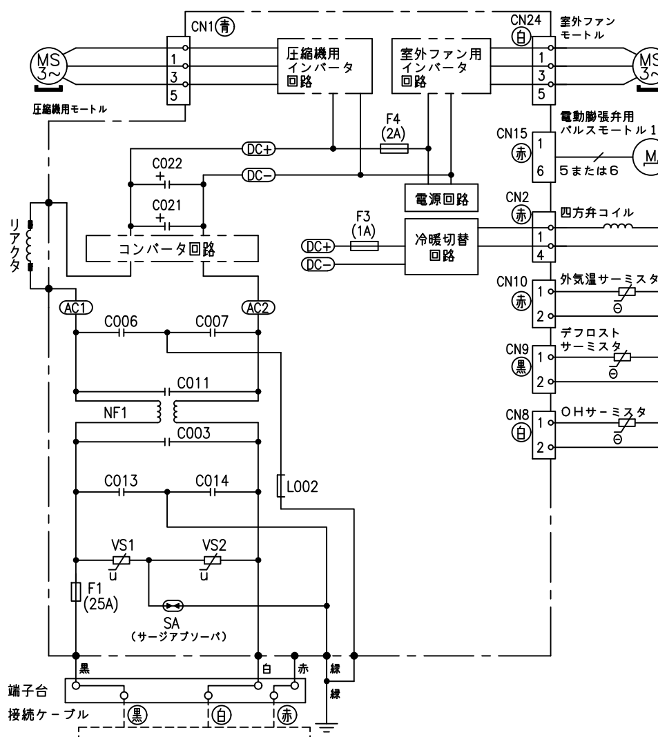
配線図 RAC-XC36L2
