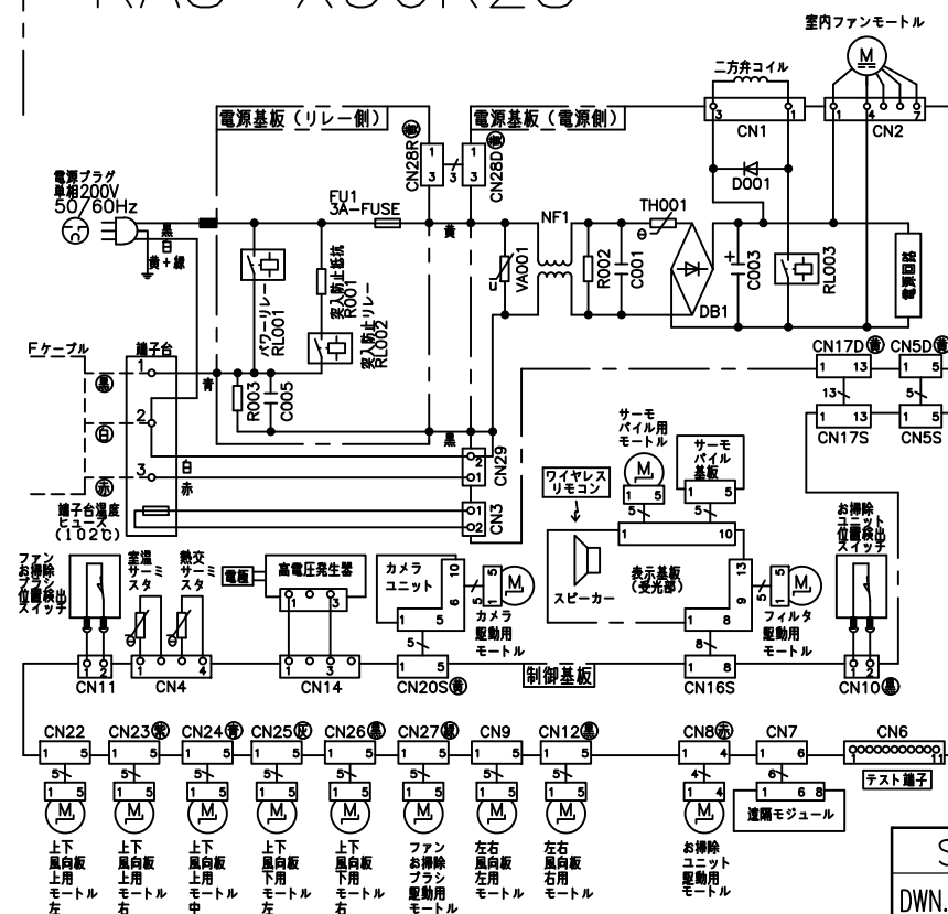
配線図 RAS-X36K2S
