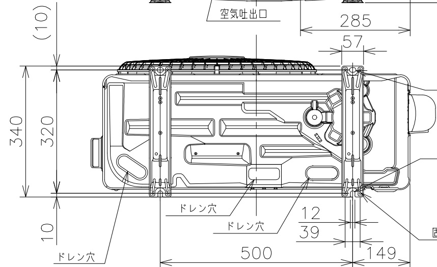
背面図
