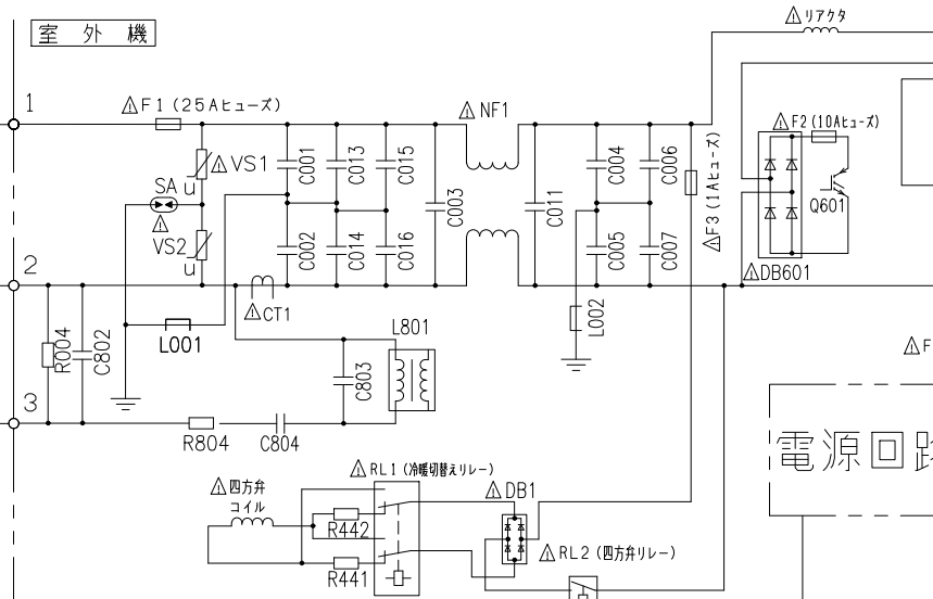
制御回路
