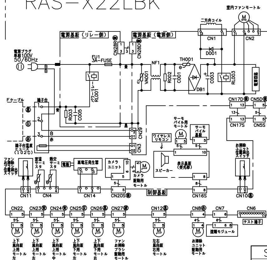
配線図 RAS-X22LBK
