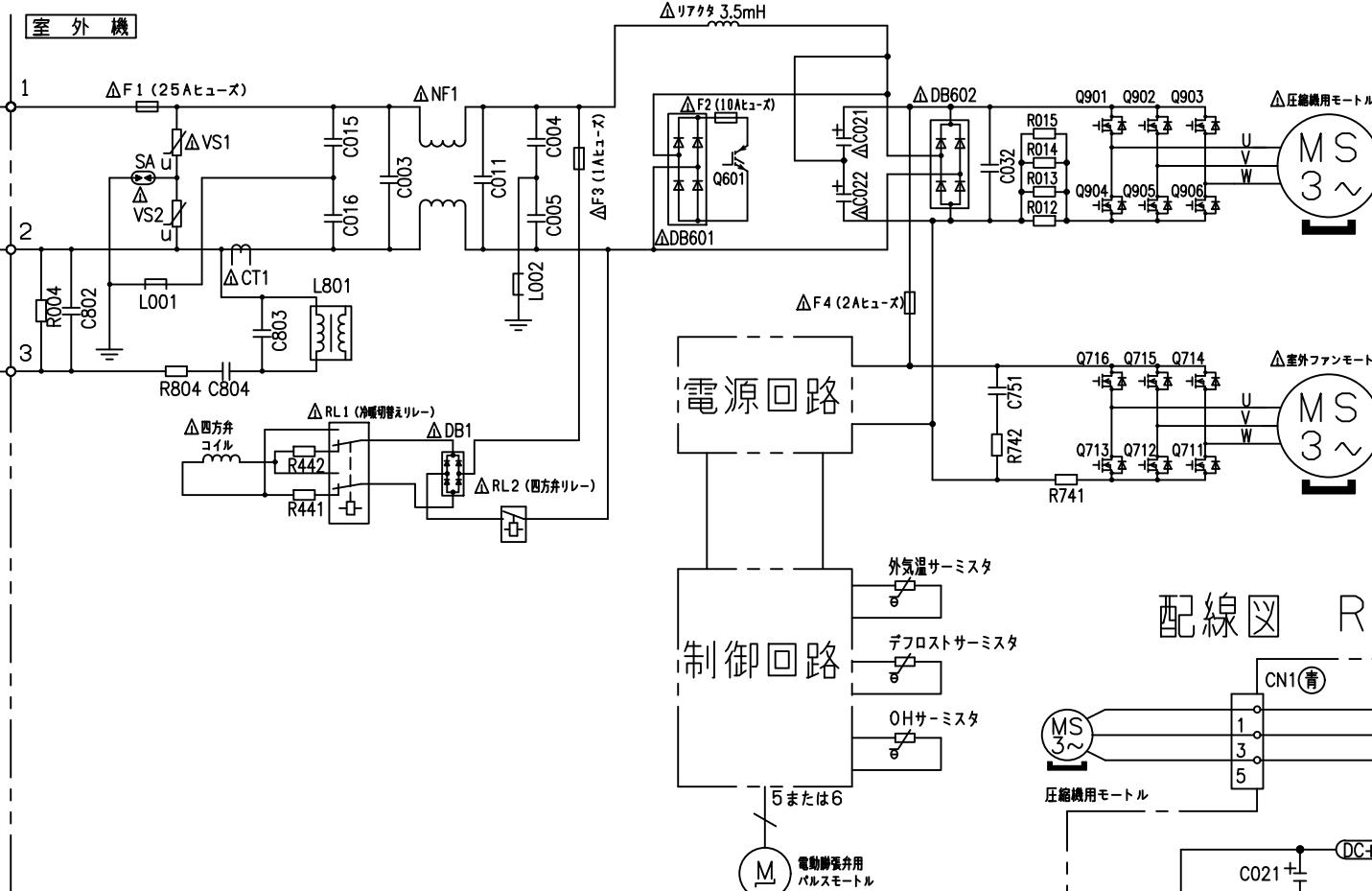
配線図 RAS-X22LBK
