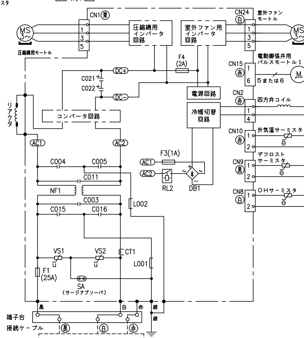
配線図 RAC-X22LBK
