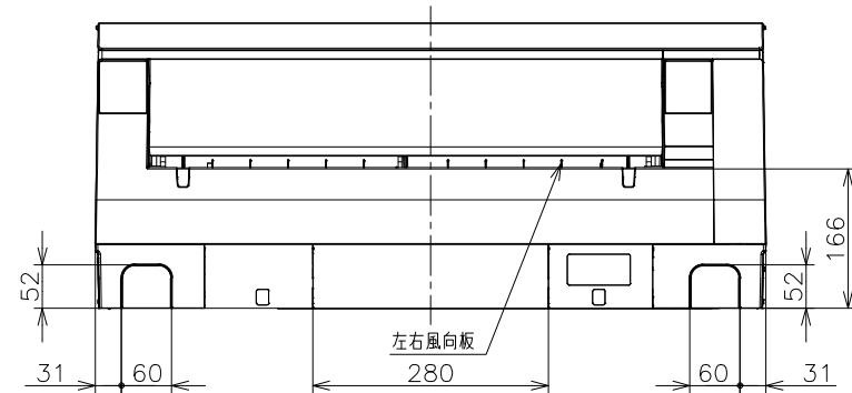
背面図
