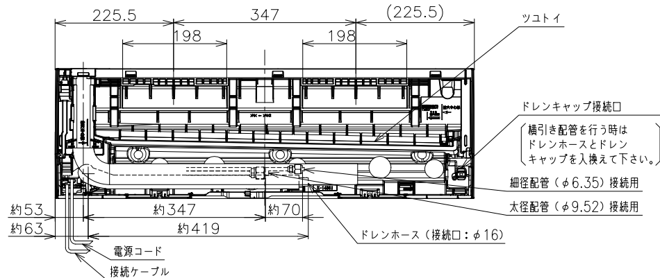
背面図
