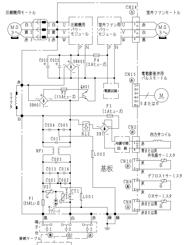
配線図 R A C - S P 4 0 B 2
