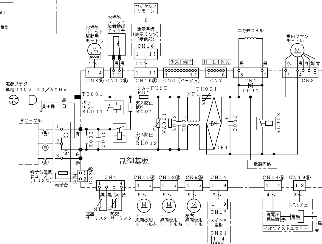
配線図 R A S - S P 4 0 B 2
