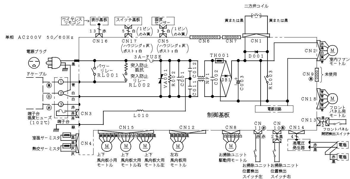
配線図 RAS-SJ40W2
