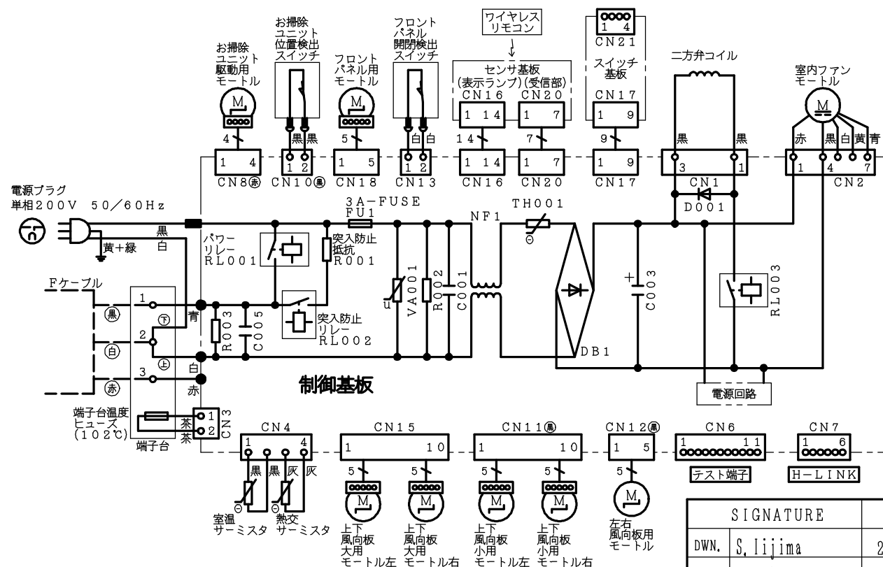
配線図 RAS-SE56E2
