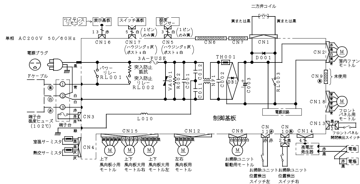
配線図 RAS-SC50W2
