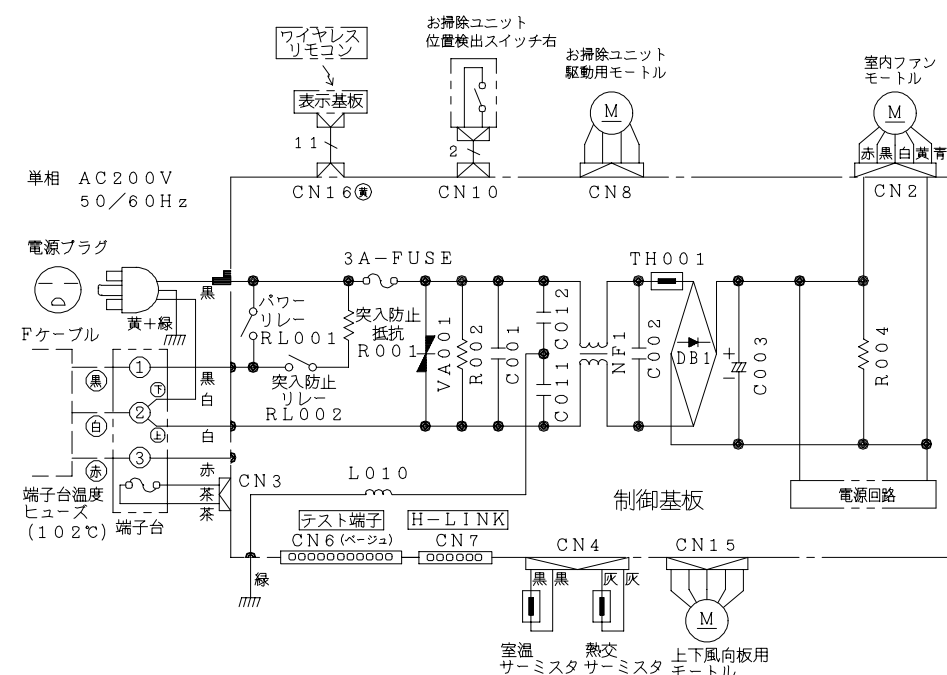
配線図 R A S - M J 5 0 X 2
