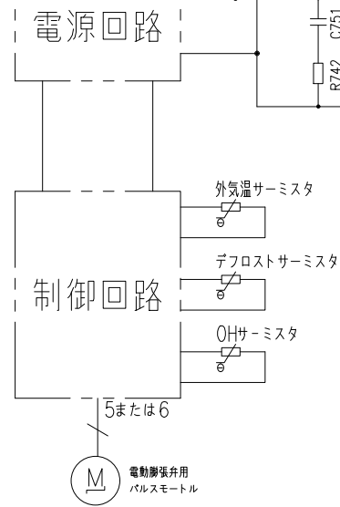
配線図 RAS-MJ25KE
