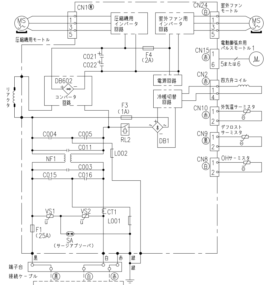
配線図 RAC-MJ25KE
