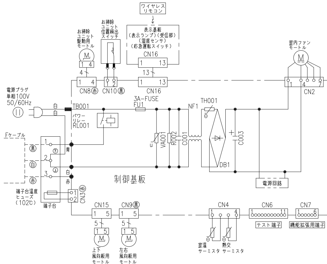
配線図 RAS-MJ25KE
