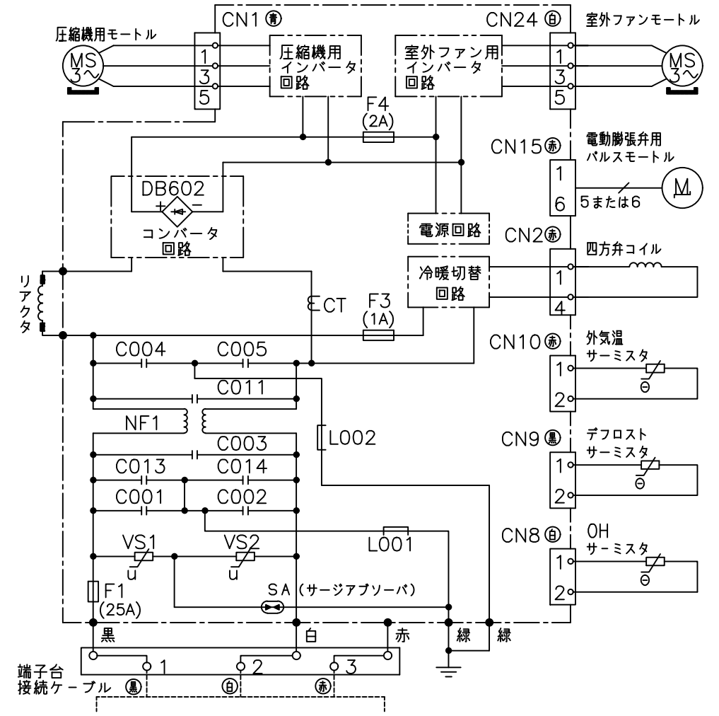
配線図 RAC-L28JE7
