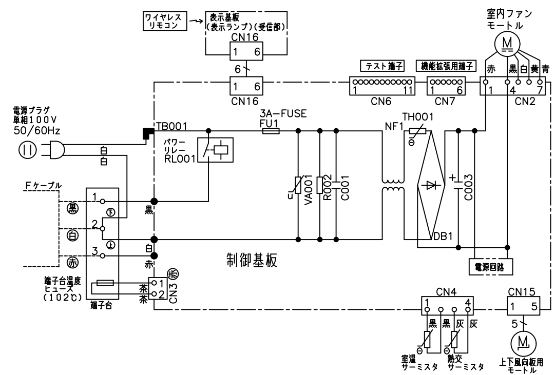
配線図 RAS-L28JE7
