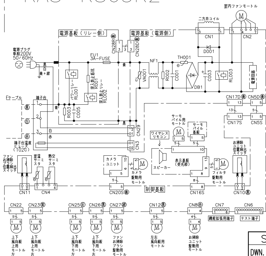
配線図 RAS-KS63K2
