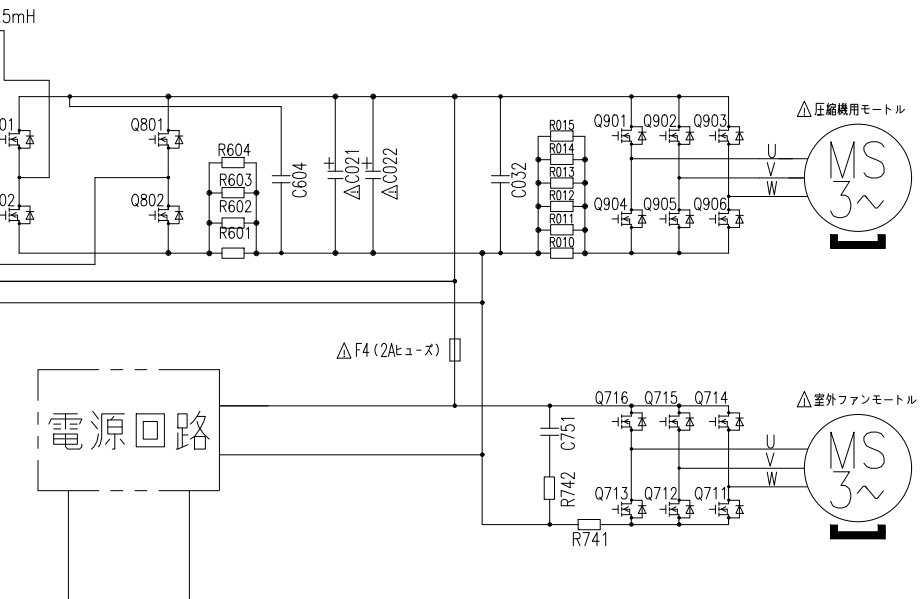
配線図 RAC-KS63K2
