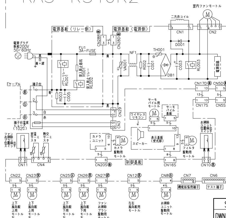
配線図 RAS-KS40K2
