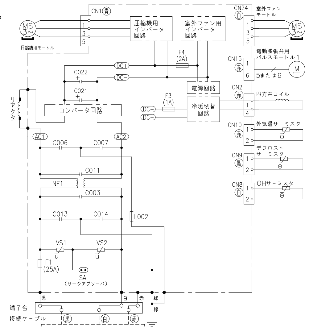
配線図 RAC-KS40K2
