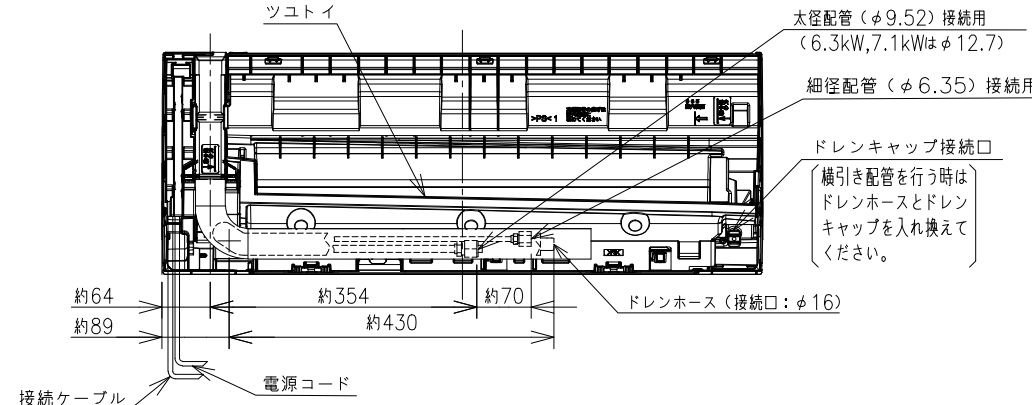
背面図
